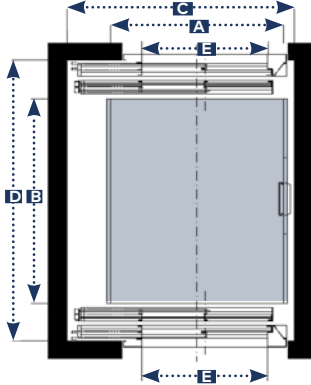
2 EMBARQUES (MECÁNICA LATERAL) ACCESO 180° PUERTAS TIPO 2HT
