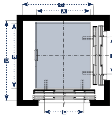
2 EMBARQUES (MECÁNICA LATERAL) ACCESO 90° PUERTAS TIPO 4HC
