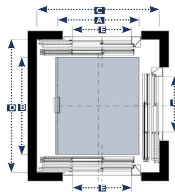
3 EMBARQUES (MECÁNICA LATERAL) ACCESO 0° PUERTAS TIPO 2HT
