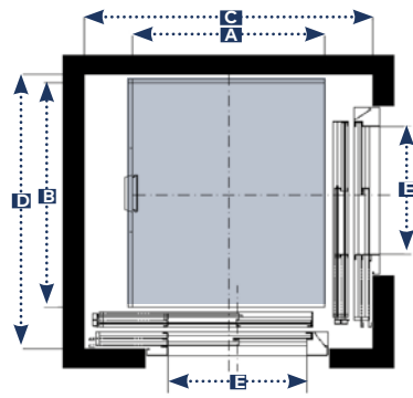
2 EMBARQUES (MECÁNICA LATERAL) ACCESO 90° PUERTAS TIPO 2HT
