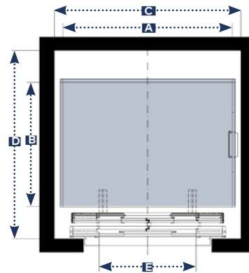
1 EMBARQUE (MECÁNICA FONDO) ACCESO 0° PUERTAS TIPO 4HC
