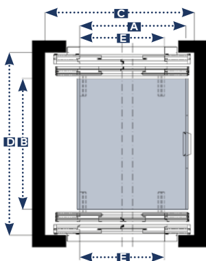
2 EMBARQUES (MECÁNICA LATERAL) ACCESO 180° PUERTAS TIPO 4HC
