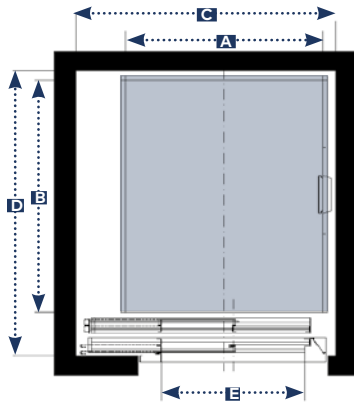
1 EMBARQUE (MECÁNICA LATERAL) ACCESO 0° PUERTAS TIPO 2HT
