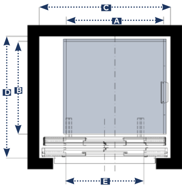
1 EMBARQUE (MECÁNICA LATERAL) ACCESO 0° PUERTAS TIPO 4HC
